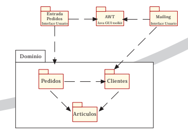
Diag. Componentes
